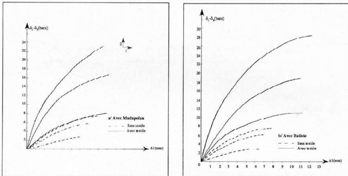
Figure 6 : Essai triaxial - limon argileux. Eprouvette recouverte latéralement.
