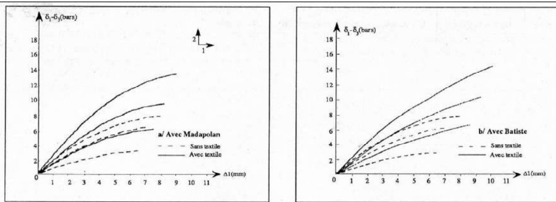
Figure 5 : Essai triaxial - limon argileux. Eprouvette recouverte à moitié.
