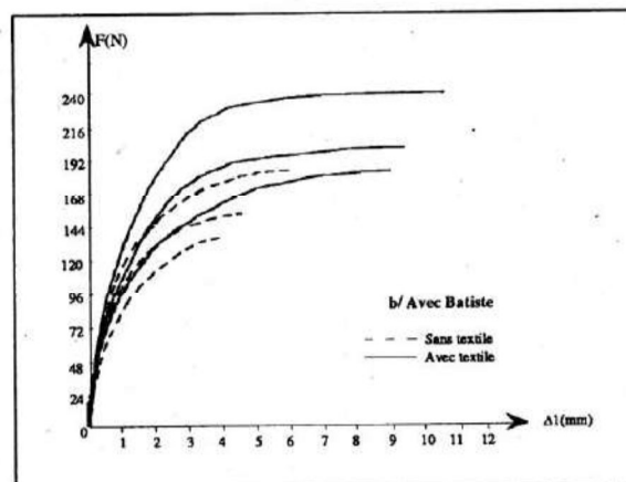
Figure 2 : Essai de Casagrande - limon argileux. Les deux demi-boîtes recouvertes.
