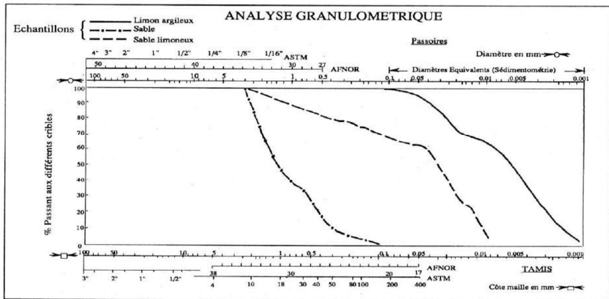
Figure 1 : Analyse granulométrique des 3 types de sols utilisés.
