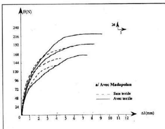
Figure 4 : Essai de Casagrande - limon argileux. Une demi-boîte recouverte.
